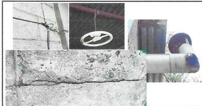
FOTO 5: EL PISO DE CONCRETO ESTÁ EN MAL ESTADO, LA CONEXIÓN ELÉCTRICA ESTÁ INSERVIBLE Y LA ESTUFA Y CHIMENEA EN MAL ESTADO POR LO QUE ES NECESARIO CAMBIAR ESTOS ELEMENTOS EN
