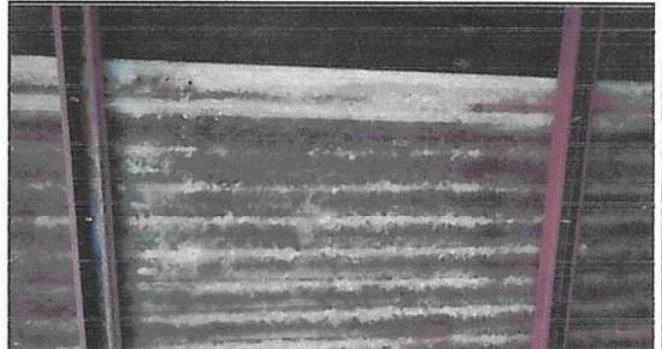
FOTO 2: EN EL TECHADO DE LA COCINA SE PUEDE OBSERVAR QUE LA ESTRUCTURA SE HA PICADO PORQUE NO TUVO CON ANTICORROSIVO, ES NECESARIO SU CAMBIO Y LAS LAMINAS QUE ESTAN PICADAS
